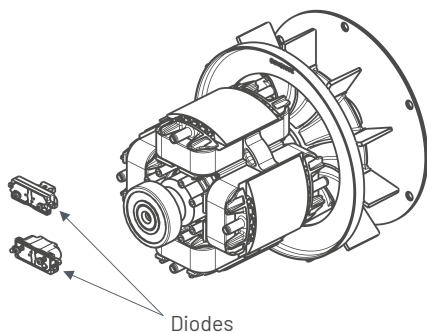
Diodes avvitati facilmente rimovibili Screwed diodes easily removable
