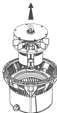
Facilità nell'estrarre il rotore Easy rotor extracting
